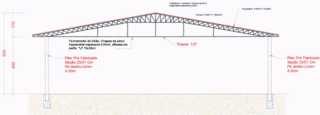
CORTE AA Escala: 1/100
