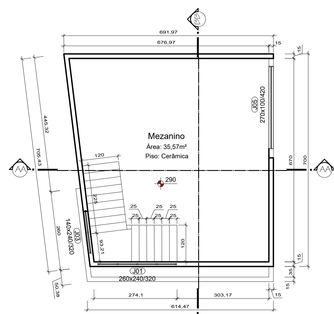
PLANTA BAIXA MEZANINO ESC: 1:75
