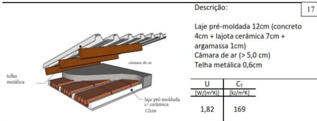
Figura 4 – Coeficientes Teto/Telhado
