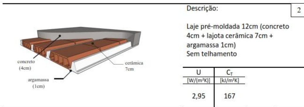
Figura 5 – Coeficientes Piso
