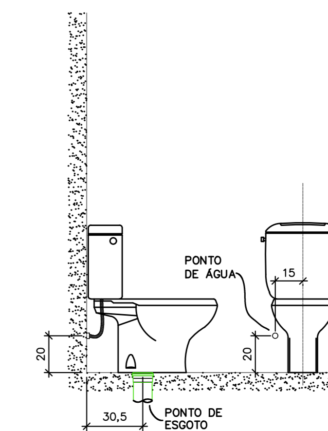
DETALHE VASO SANITÁRIO
