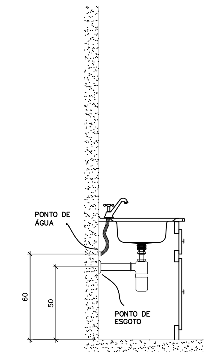
DETALHE PIA DE COZINHA TORNEIRA DE BANCADA
