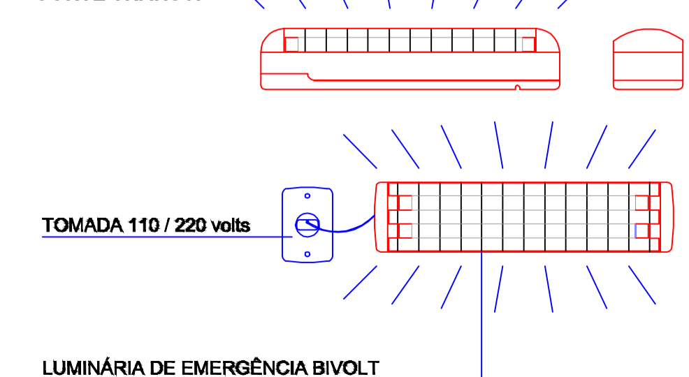
DETALHE - ILUMINAÇÃO DE EMERG. S/ESC.
