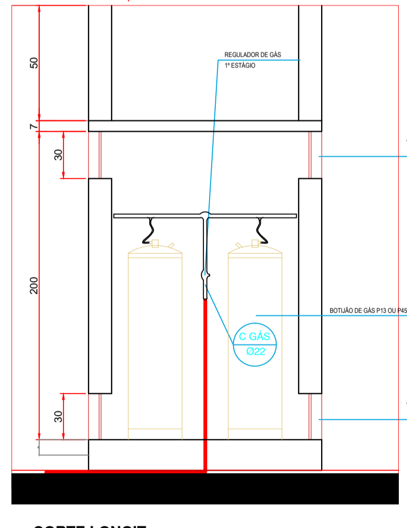
CORTE LONGIT.
