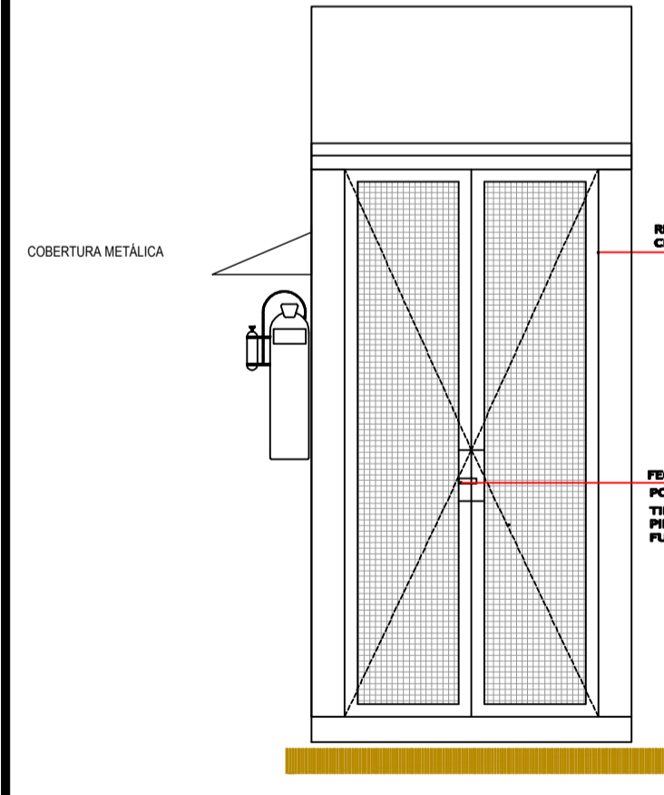
ELEVAÇÃO 01
