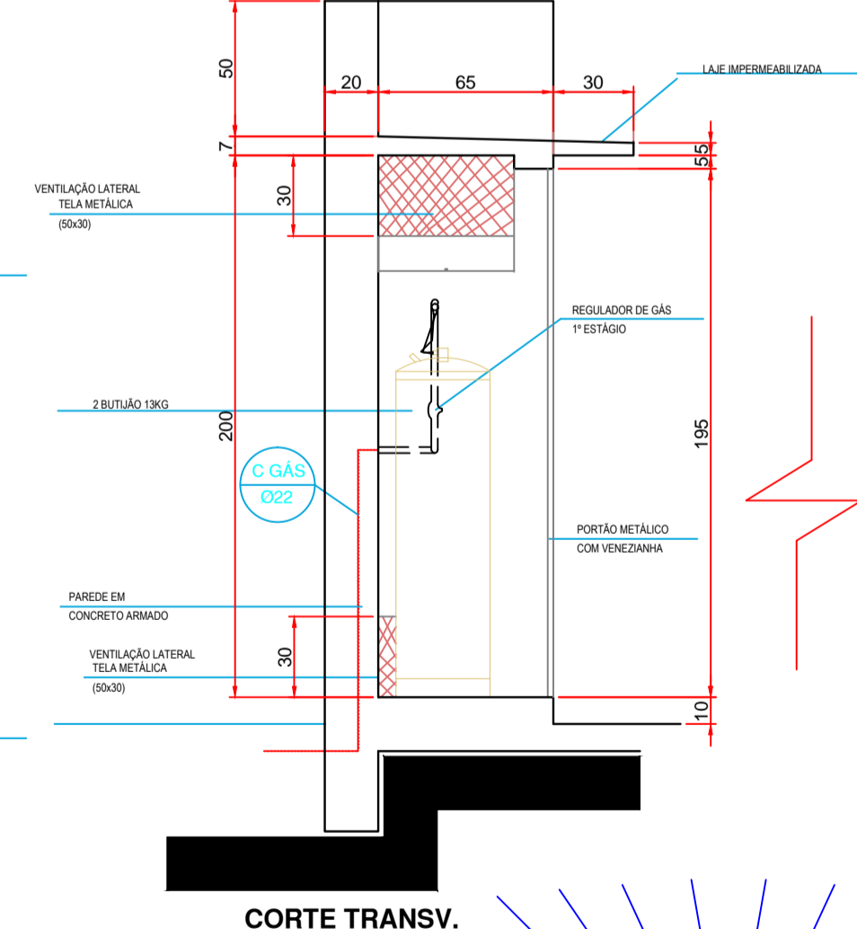
CORTE TRANSV.
