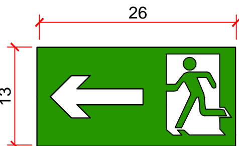
PLACA DE INDICAÇÃO DO SENTIDO SAÍDA ESQUERDA ESCALA: 1:15
