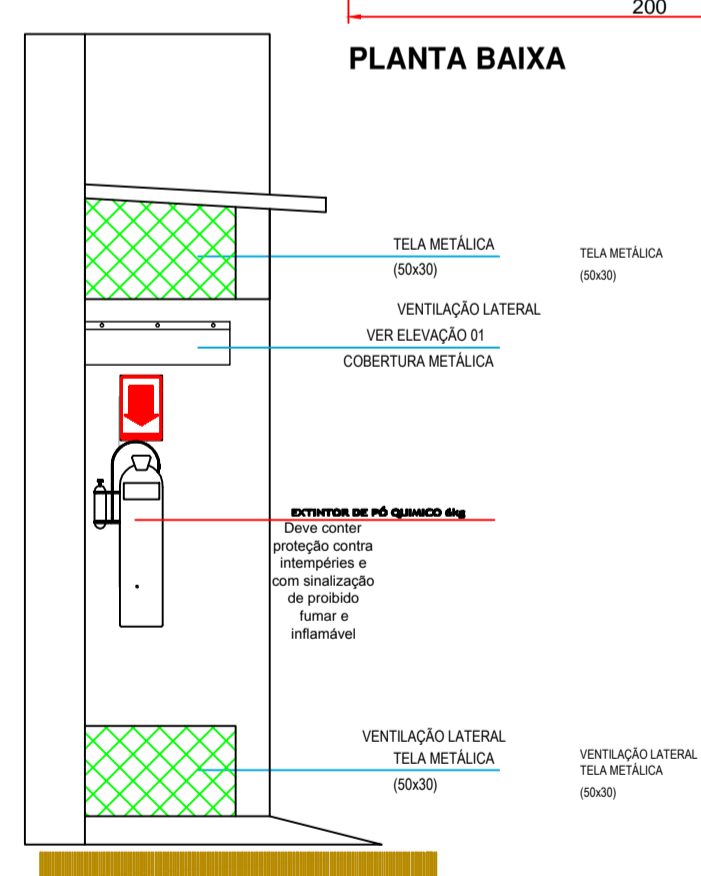
ELEVAÇÃO 02
