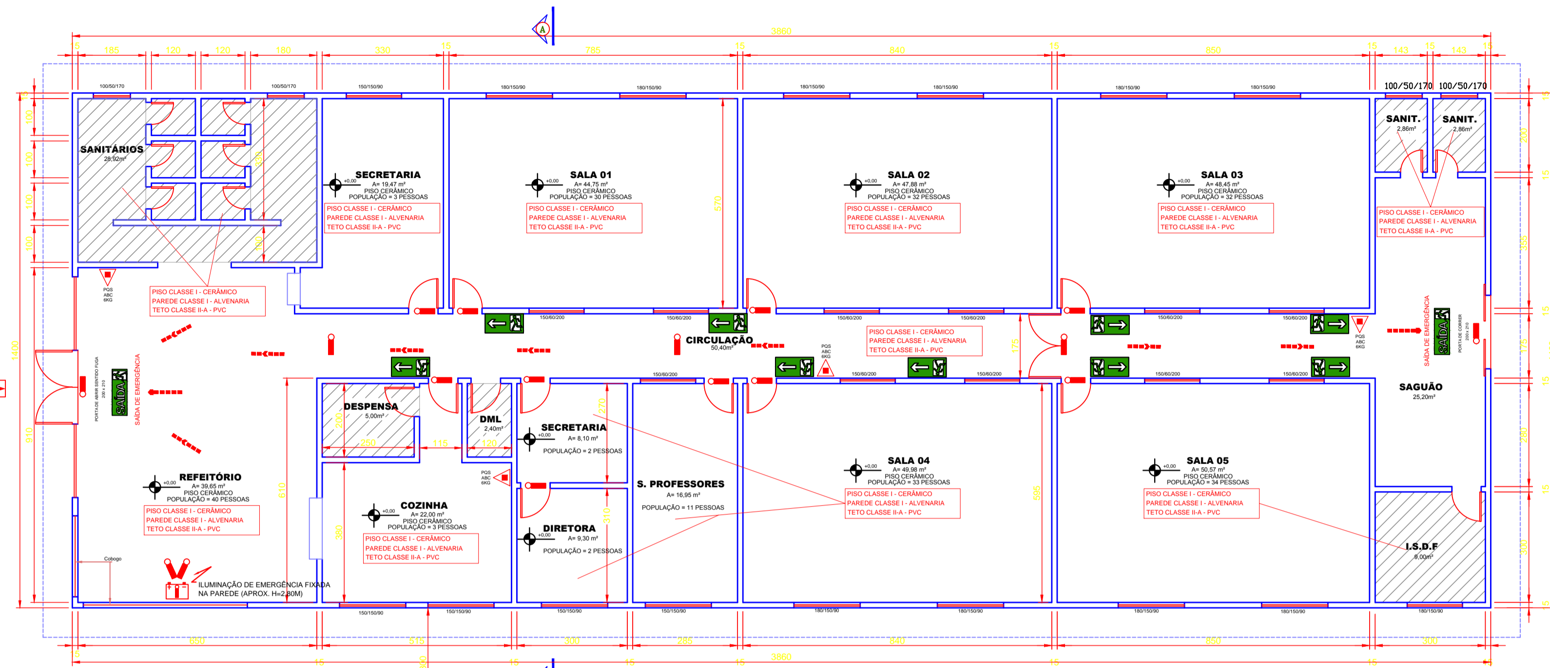
PLANTA BAIXA ESCALA: 1/70 Área: 540,40m 2
