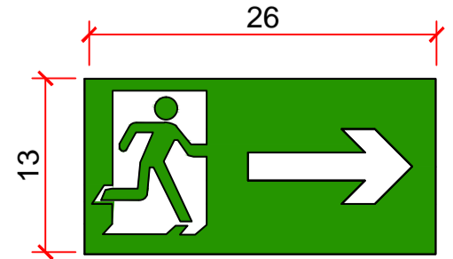
PLACA DE INDICAÇÃO DO SENTIDO SAÍDA DIREITA ESCALA: 1:15
