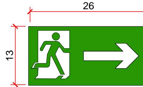
PLACA DE INDICAÇÃO DO SENTIDO SAÍDA DIREITA ESCALA: 1:15
