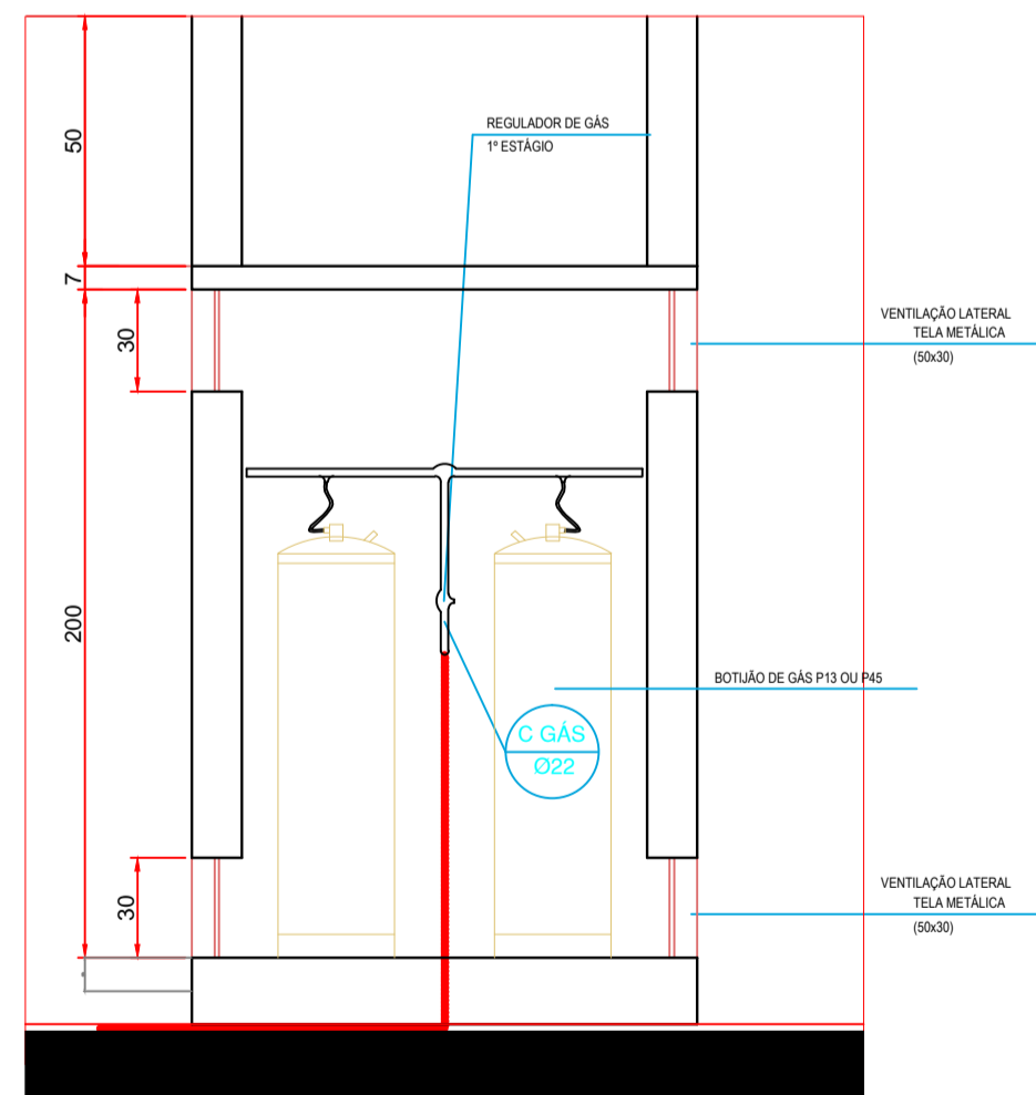
CORTE LONGIT.
