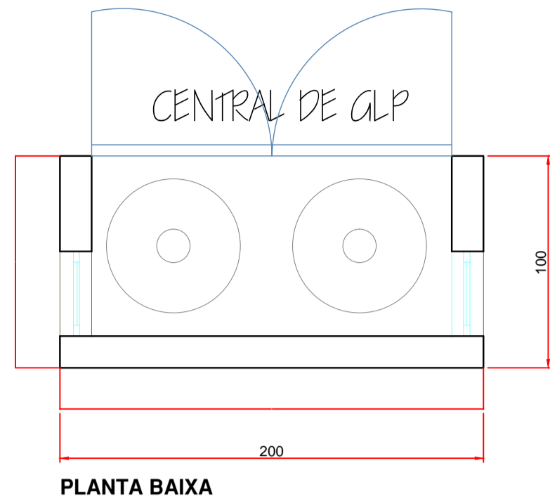
PLANTA BAIXA
