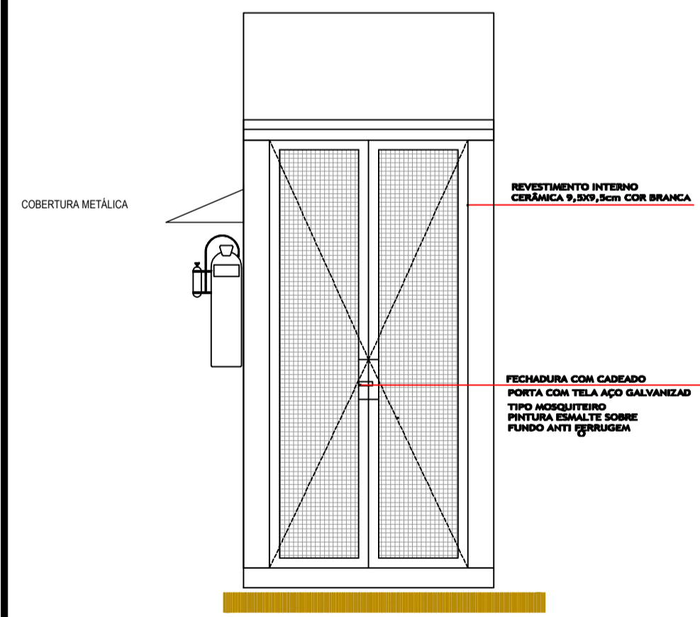
ELEVAÇÃO 01
