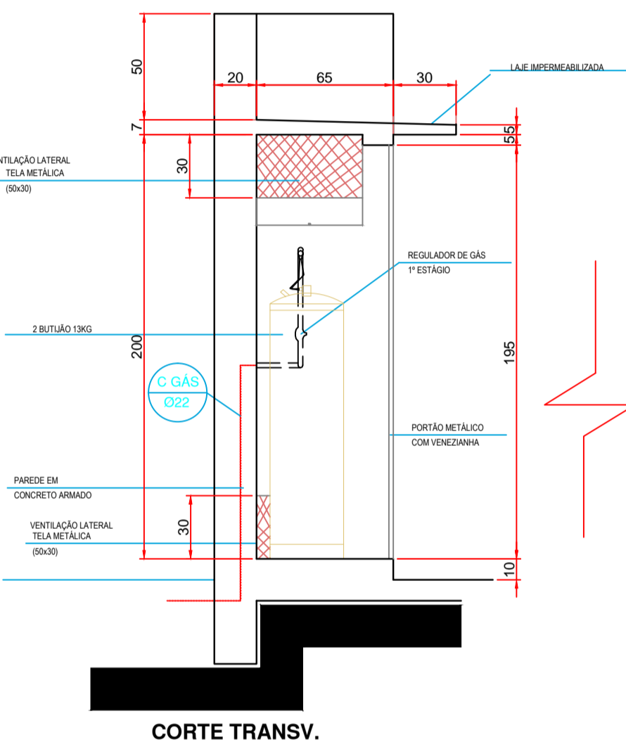
CORTE TRANSV.
